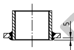
Entlüftungs-u. Ablaßmuffe innen bündig
