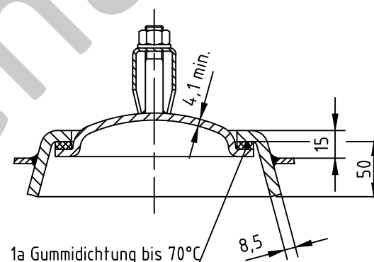
OAB 51 - Handlochverschluß 100/150 bauteilgeprüft
